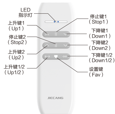
JCHR35W3A7—单通道双路
